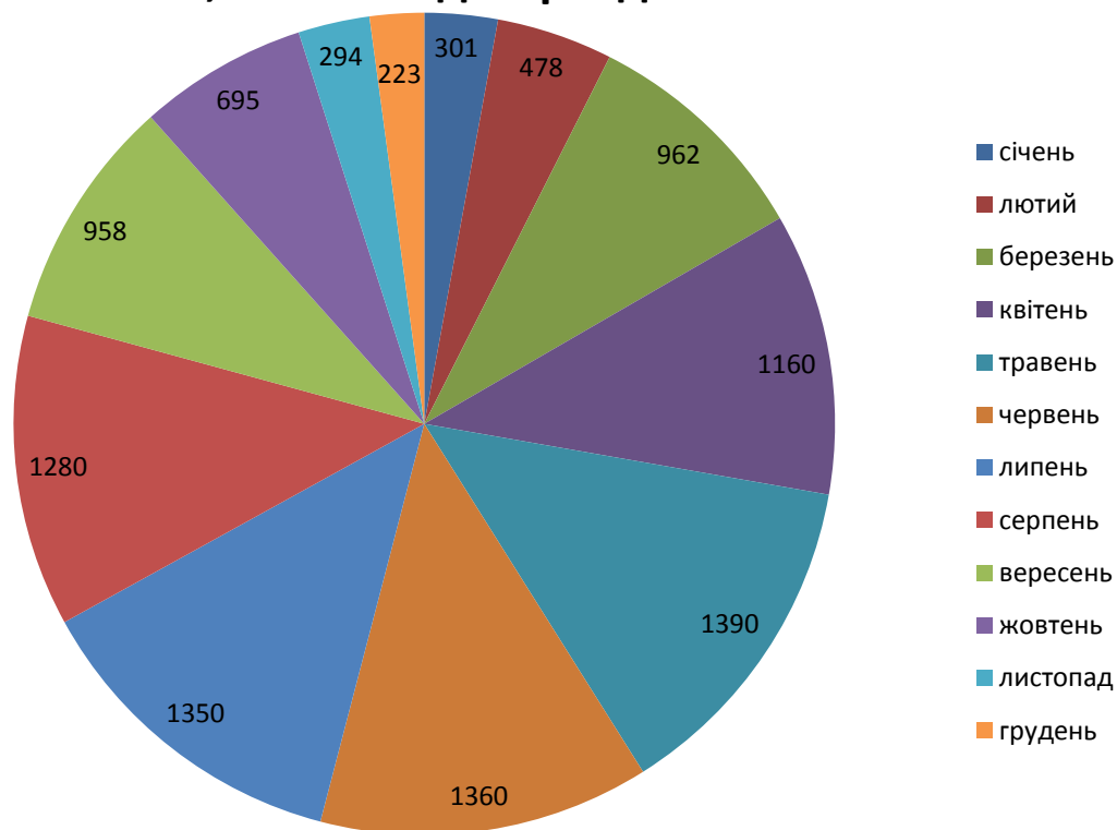
Генерація електроенергії сонячною станцією потужністю 10кВт протягом року (енерговиробіток кВт · год. по місяцях)
